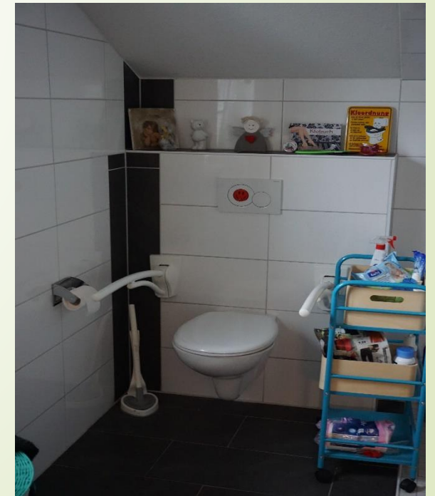
Rollstuhlgerechtes Bad nach DIN 18040
